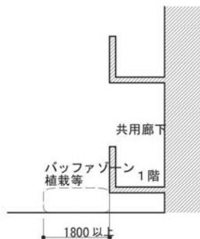
【図 離隔距離等の確保の例】
